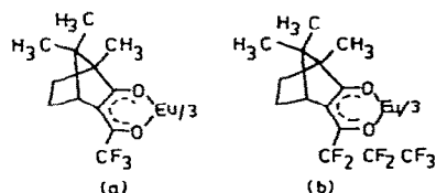
Fig. 22. Europium 1,3-diketonates.
